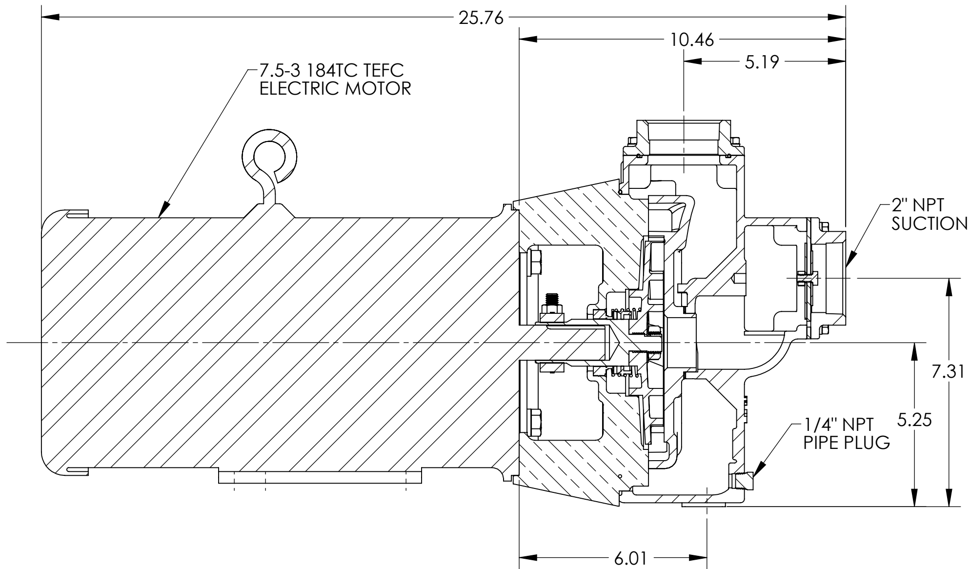
SECTION A-A
